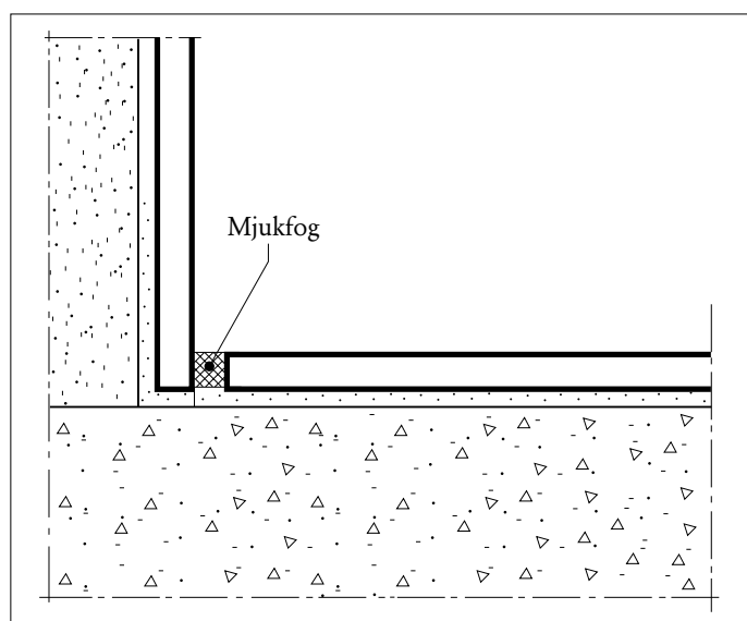
4. Mjukfog CC Höganäs Habenit 53 alt. Habenit 54 vid anslutning vägg.
